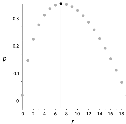
Figura 5. Valors p(20, r) per r = 0, 1, \dots, 19 .
