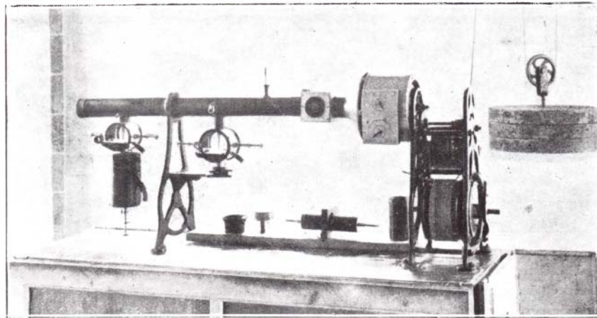
Fig. 13 Aparell de Gardien per a l'estudi dels ions
