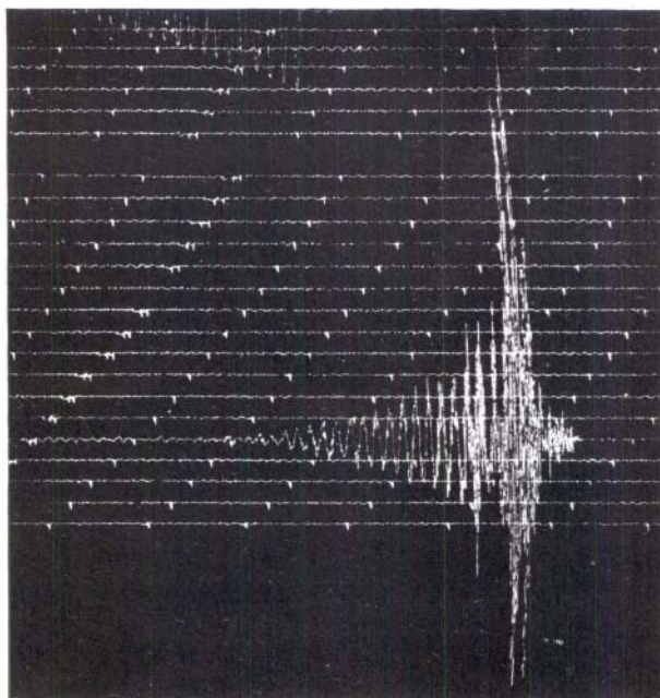
II.—Gràfica del pèndol de 150 quilos
