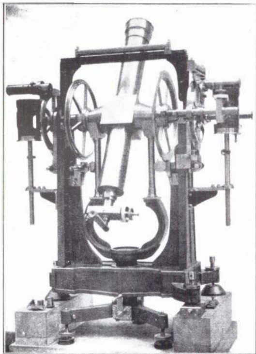
Fig. 24 Cercle meridià de l'Observatori de l'Ebre
