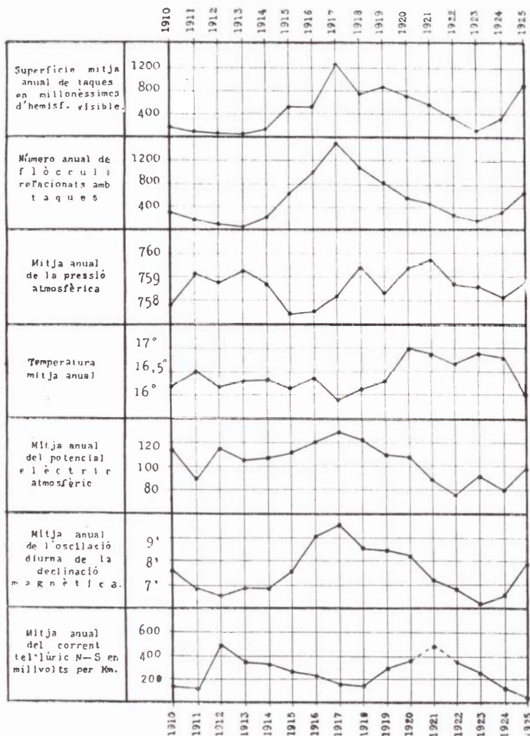
Fig. 25 Correl·lació entre els principals fenòmens registrats a l'Observatori de l'Ebre, d'ençà de la publicació del seu butlletí mensual (1910-1925)
