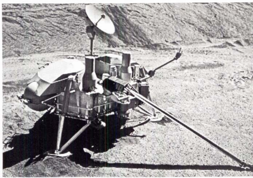
Projecte Viking: model de les naus espacials enviades a Mart (Font: NASA)
