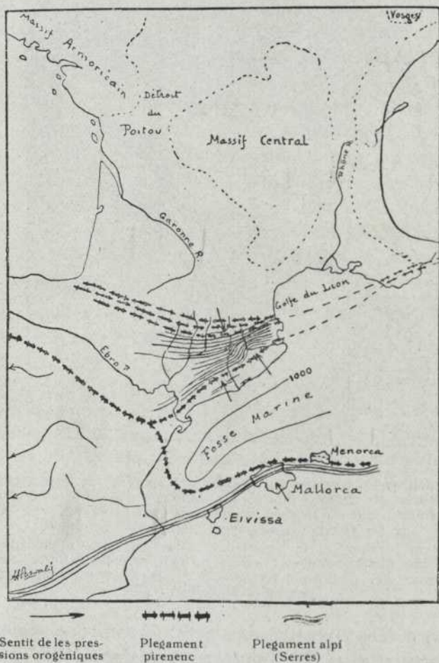
Fig. 9 Esquema dels plegaments terciaris a Catalunya, conca de l'Ebre i Balears. Remarqui's la superposició dels plegaments pireneics i dels plegaments alpins
