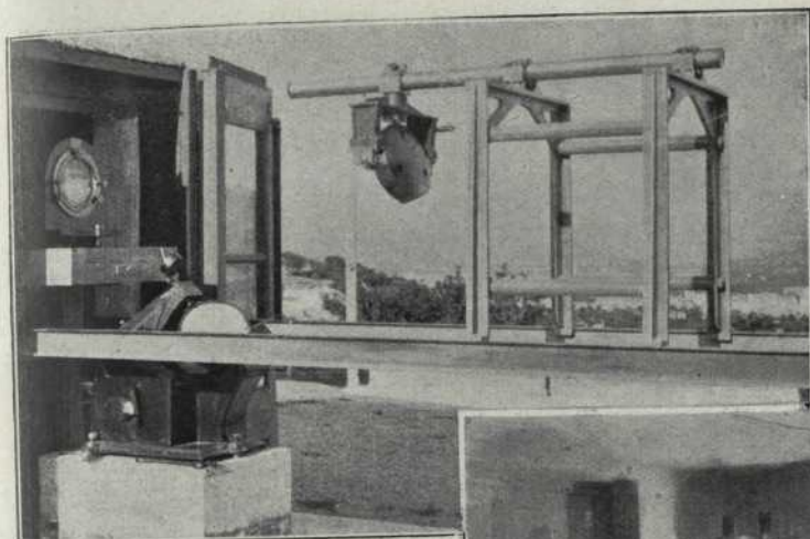
Fig. 5 Telescopi horitzontal amb ce- losttat Grubb de l'Observatori de l'Ebre
