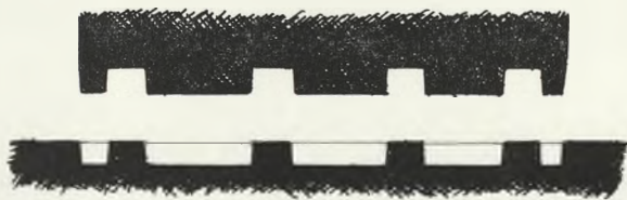
Figura 4. — Alçat per la secció A-B. A dalt, secció del punxó. A baix, secció de l'impromta sobre el metall.
