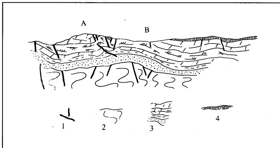
Tall transversal del solc de Juncosa (Mapa geològic d'Espanya, 1/50.000 Valls).
