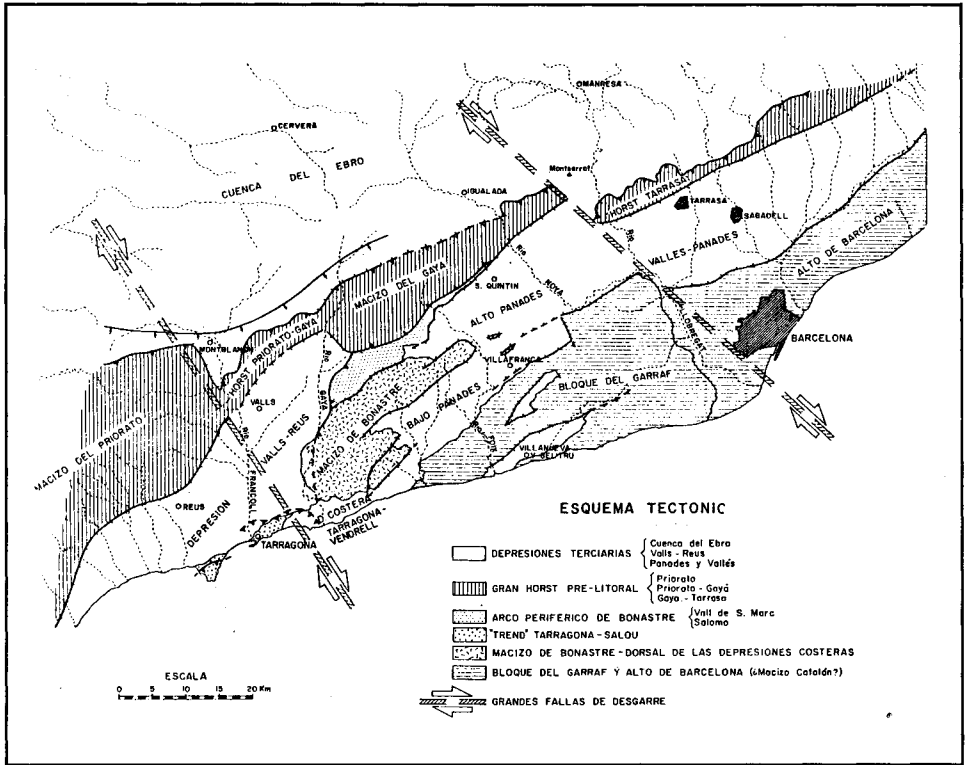
(GRAVAT: L'ESQUEMA TECTÒNIC)
