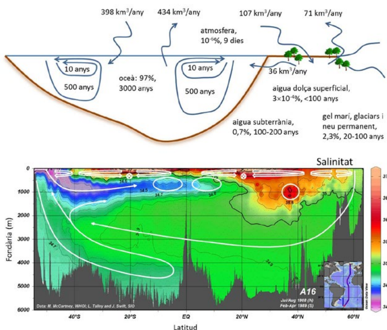
↑ Figura 1. (Superior) Fracció d'aigua (%) i temps de residència (anys) en els diferents compartiments de la Terra, així com els fluxos (km³/any) més rellevants entre aquests compartiments. El volum total d'aigua al planeta és d'uns 1,4 \times 10^9 \text{km}^3 . (Inferior) Distribució de la salinitat a l'oceà Atlàntic, en funció de profunditat i latitud, al llarg del traçat que es mostra al requadre interior (WOCE-ATLAS, 2017). Les condicions atmosfèriques són les que determinen la salinitat de cada massa d'aigua en origen, prop de la superfície dels oceans: les línies dobles il·lustren el circuit pulmonar (termoclí, amb un origen relativament proper) i les línies senzilles figuren part del llarg circuit sistèmic (circulació global profunda).
