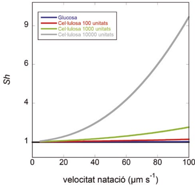
↑ Figura 2. Comportament del Sh amb la velocitat de natació d'un bacteri de 0,5 \mu\text{m} de diàmetre. Les línies corresponen a diferents compostos de creixent pes molecular i, per tant, de decreixent difusivitat. La línia horitzontal negra marca Sh = 1 (difusió molecular només).
