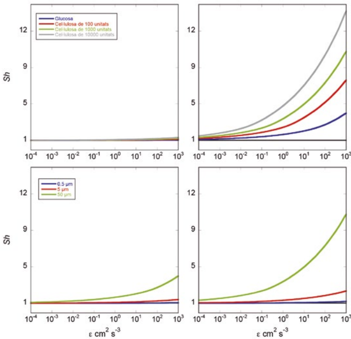
↑ Figura 3. Comportament del Sh amb la turbulència per a diferents compostos de creixent pes molecular i, per tant, de decreixent difusivitat (dalt) per a un microorganisme de 0,5 \mu\text{m} de diàmetre (dalt-esquerra) i 50 \mu\text{m} de diàmetre (dalt-dreta), i per a diferents mides de microorganismes (baix) per a glucosa (baix-esquerra) i per a cel·lulosa de 1.000 monòmers (baix-dreta). La línia horitzontal negra marca Sh = 1 (difusió molecular només).
