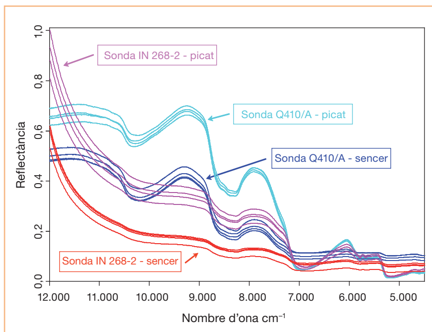
FIGURA 2. Espectres originals obtinguts amb les dues sondes i amb les dues presentacions.
