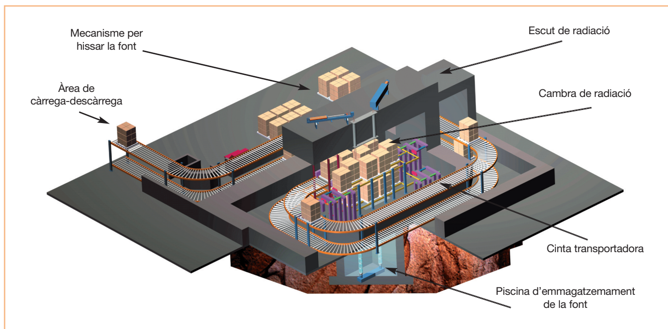
FIGURA 2. Planta d'irradiació amb cinta transportadora de palets.
