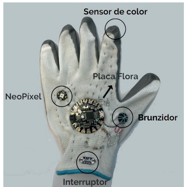
FIGURA 14. Guant que detecta colors i els converteix en sons que va ser dissenyat per uns estudiants del grau en tecnologies industrials. FONT: Arxiu dels autors.
