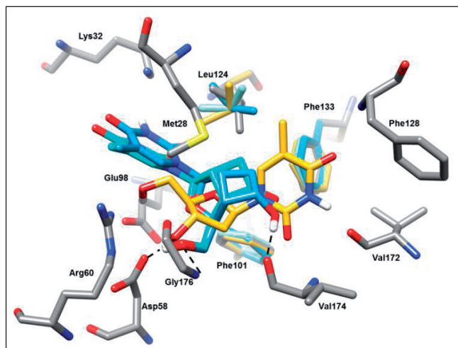
FIGURA 7. Anàleg 5 (cian) superposat amb 6 (blau) i dT (groc) en el lloc actiu de la TK1 (els residus provinents de l'estructura de raigs X es mostren en gris). Els enllaços de pont d'hidrogen es mostren amb una línia discontinua.
