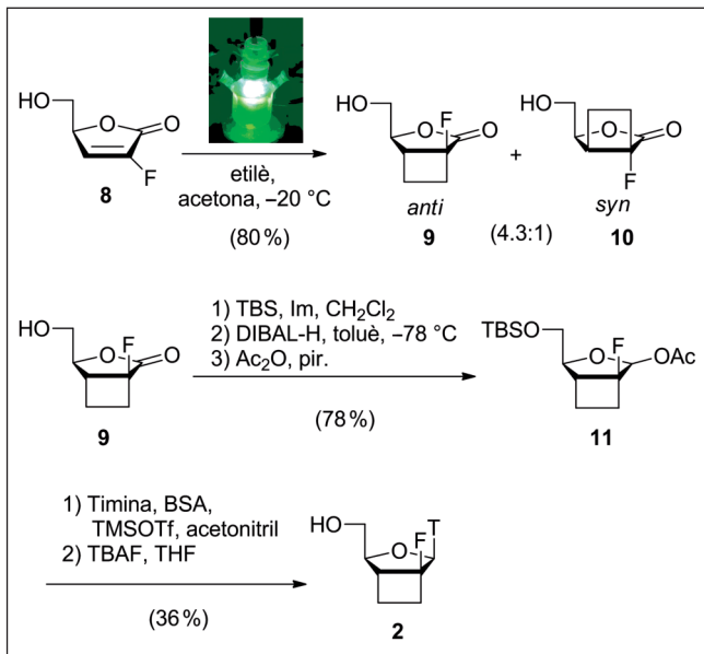
FIGURA 4. Exemple de preparació dels anàlegs conformacionalment rígids. Síntesi de l'anàleg fluorat 2.
