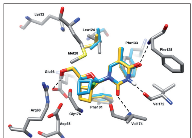
FIGURA 6. Anàleg 3 (groc) superposat amb 1 (blau) en el lloc actiu de la TK1 (els residus provinents de l'estructura de raigs X es mostren en gris). Els enllaços de pont d'hidrogen es mostren amb una línia discontinua.
