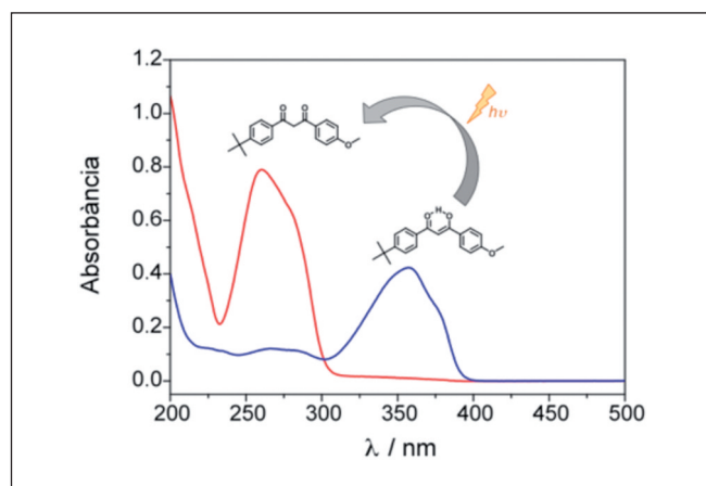
FIGURA 4. Espectres d'absorbància de la BM-DBM(E) i la BM-DBM(K)-Me (avobenzona metilada en la posició \alpha del carbonil). S'ha utilitzat aquesta darrera espècie per mesurar les propietats l'avobenzona cetònica, ja que fixa el tautòmer dicetònic.
