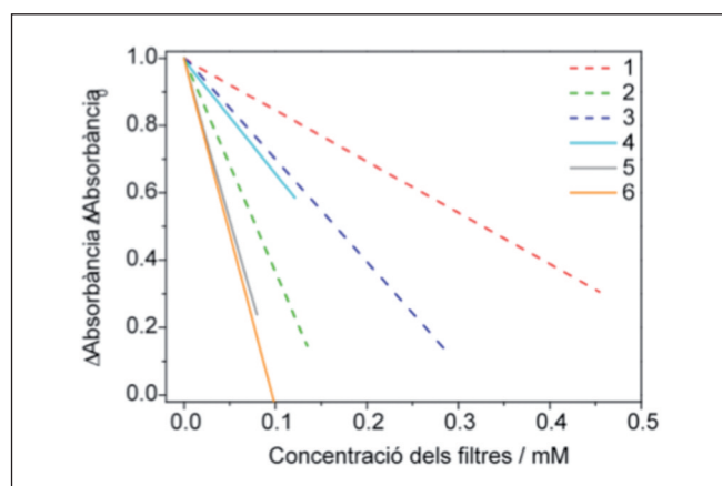
FIGURA 8. Amplituds normalitzades dels senyals de la ^3\text{BM-DBM(K)-Me} en presència dels diferents filtres UV (1-6) en funció de la concentració d'aquests. La normalització està referida al senyal inicial en absència de filtre.
