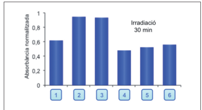
FIGURA 10. Descomposició dels diferents filtres UV fotosensibilitzats per acetona. Els valors d'absorbància relativa que es presenten fan referència a 30 min d'irradiació del sistema.
