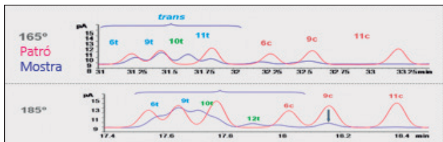
FIGURA 9. Superposició de cromatogrames: el blau correspon a l'extracte de la fracció trans obtingut per fraccionament per LC amb microcolumna d'ió plata (Supelco), i el de color vermell és del patró « cis-trans FAME Mix». En els registres s'ha ampliat la zona d'interès. Els cromatogrames superiors s'han registrat en mode isotèrmic a 165 °C i els cromatogrames inferiors s'han registrat en mode isotèrmic a 185 °C.
