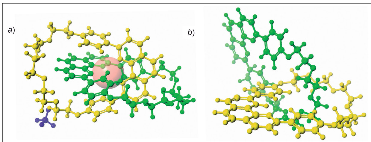
FIGURA 2. Estructures de raigs X a) del metal·lo-[2]catenà i b) del [2]catenà. Els macrocicles entrecreuat es representen com a models de boles i barres en dos colors diferents per facilitar la seva visualització. El Cu(I) en a) es mostra com a model CPK.
