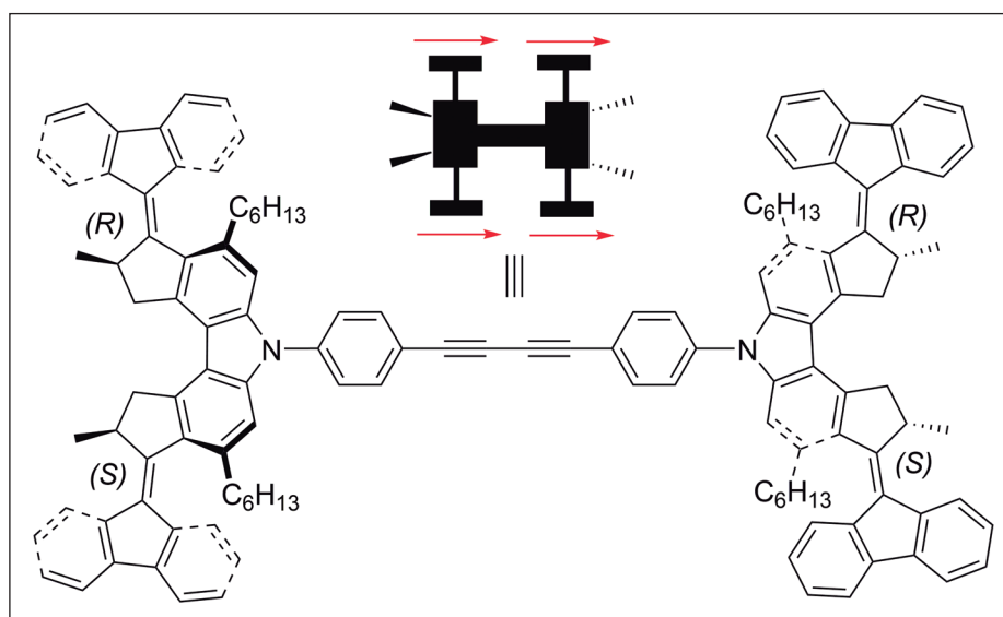
FIGURA 10. Estructura molecular de l'isòmer meso-( R,S,R,S ) del nanotxe desenvolupat per Feringa i els seus col·laboradors.
