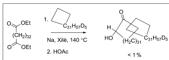
ESQUEMA 1. Síntesi estadística d'un [2]rotaxà.
