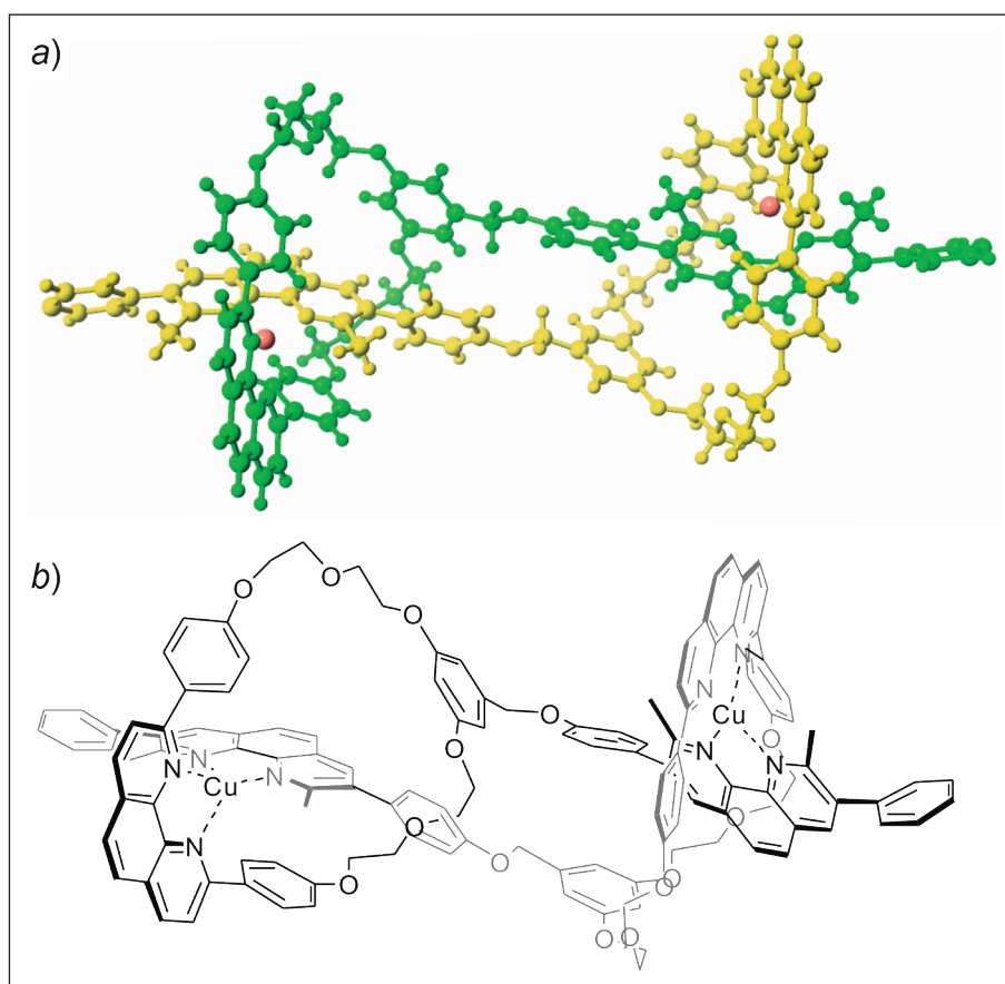
FIGURA 8. a) Estructura de raigs X d'un metallo-[2]daisy chain; b) estructura molecular corresponent.
