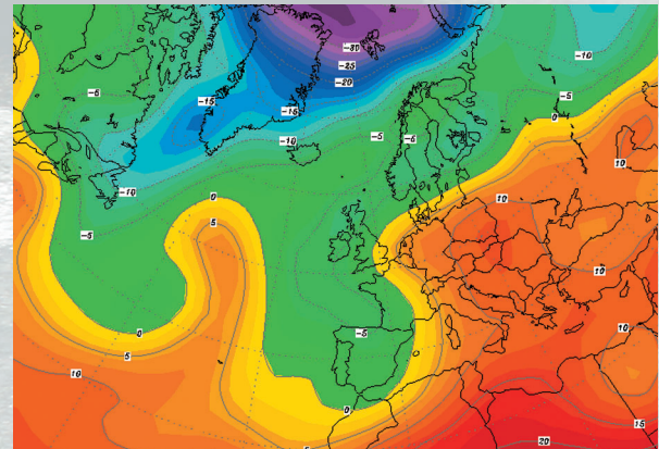
Situació atmosfèrica del 8 d'abril de 1986, que va ser més fred del normal a Espanya. A l'esquerra, situació a uns 5.500 metres d'altitud, i a la dreta, temperatures a uns 1.500 metres d'altitud. El sector en verd mostra l'entrada d'aire polar que va afectar Espanya en ple mes d'abril.
