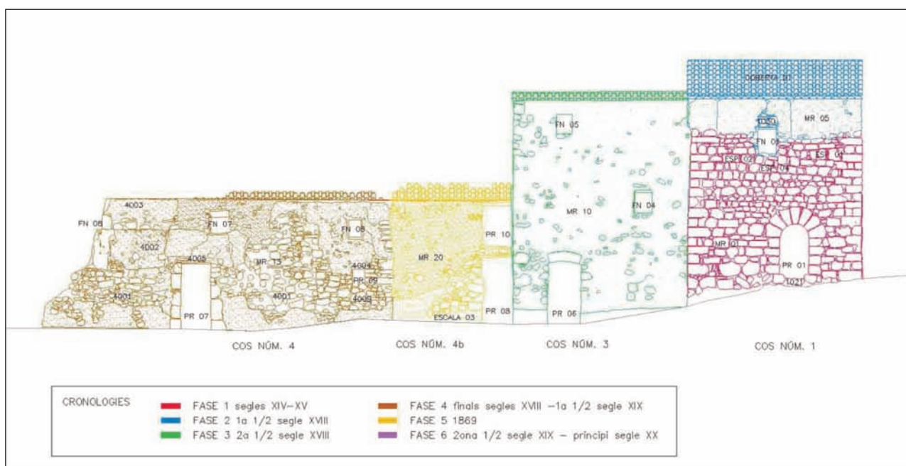
FIGURA 5. La identificació i registre dels paraments i elements parietals d'un conjunt arquitectònic són un document gràfic essencial per poder analitzar, interpretar i identificar la seqüència de l'evolució constructiva que ha experimentat aquesta arquitectura al llarg del temps. (Estudi històric i arquitectònic del mas Vidal, a les Pobles, Aiguamúrcia. Marina Miquel i Isidre Pastor, 2007.)
