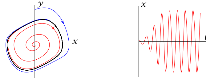
FIGURA 1: A l'esquerra, un cicle límit al pla (x, y) i dues òrbites que hi tendeixen. A la dreta, la primera coordenada x = x(t) de l'òrbita que tendeix al cicle límit des del seu interior.
