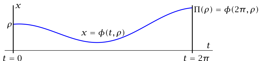
FIGURA 2: Aplicació de Poincaré.
