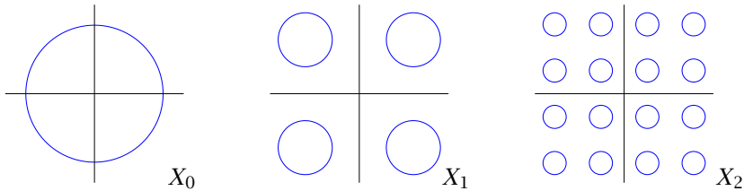
FIGURA 4: Dos passos del procés, començant amb el camp X_0 amb un únic cicle límit. Els camps X_1 i X_2 tenen quatre i setze cicles límit, respectivament.
