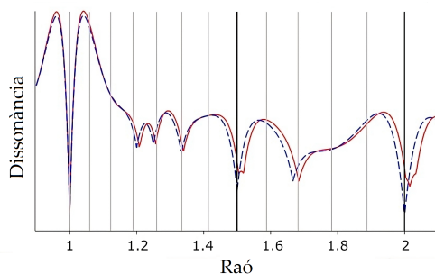
FIGURA 11: Comparació entre les corbes de dissonància d'un espectre harmònic (línia discontinuada) i de l'espectre d'una corda amb rigidesa com la del piano (línia contínua). Les línies grises verticals marquen la distribució de les notes d'una escala de temperament igual; la quinta justa i l'octava les hem marcat amb línies verticals més gruixudes perquè es puguin distingir més bé.
