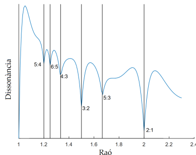
FIGURA 9: Disposició dels intervals purs a la gràfica de dissonància. S'observa que coincideixen amb els mínims de la funció de dissonància.
