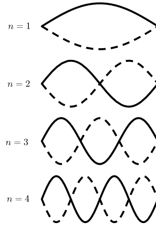
FIGURA 2: Els 4 primers modes de vibració d'una corda fixada pels extrems.
