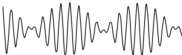
FIGURA 6: Dues ones simples superposades.
