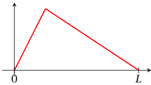
FIGURA 1: Condició inicial no diferenciable però perfectament admissible des d'un punt de vista físic.
