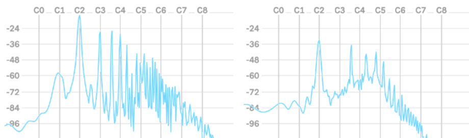
FIGURA 3: L'espectre de dos instruments que estan tocant la mateixa nota, un do d'aproximadament 130 Hz de freqüència (C2 en notació anglosaxona). L'eix horitzontal dels gràfics representa les freqüències en escala logarítmica; l'inici de cada octava està marcat amb les línies verticals. L'eix vertical representa l'amplitud mesurada en decibels. En el segon gràfic es pot veure que només apareixen els harmònics senars.
