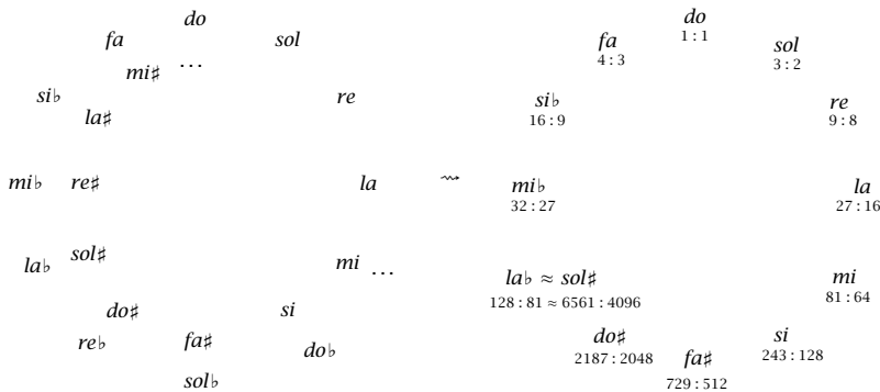
FIGURA 5: A la figura s'observa com tancar l'espiral de quintes (panell de l'esquerra) per obtenir el cicle de quintes (panell de la dreta, on hem fet explícites les raons dels intervals respecte do ). En aquest cas, la freqüència del sol\sharp (amb raó 6561 : 4096 ) baixa per tal de ser igual a la freqüència del la_b (amb raó 128 : 81 ).
