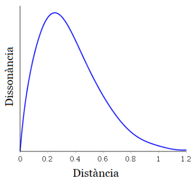
FIGURA 7: Dissonància de dos tons purs com a funció de la seva distància (mesurada en tons temperats).
