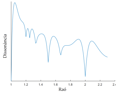
FIGURA 8: Corba de dissonància per a notes amb sis harmònics (tots amb la mateixa amplitud).
