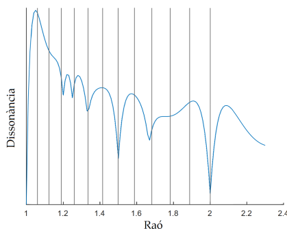
FIGURA 10: Disposició de les notes de l'escala temperada a la gràfica de dissonància.
