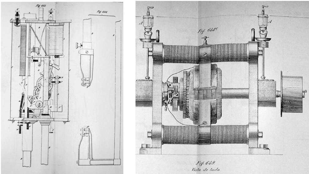
Figura 1. A l'esquerra, la làmpada Puydt i, a la dreta, la màquina Gramme L5.
