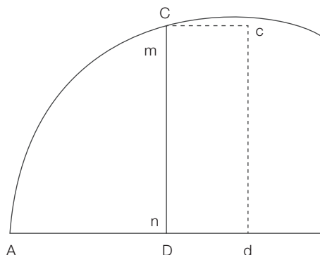
Fig. 1: La fluxió d'una superfície curvilínia.
