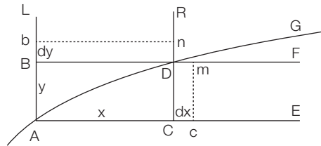
Fig. 3: La fluxió del producte de dues variables.
